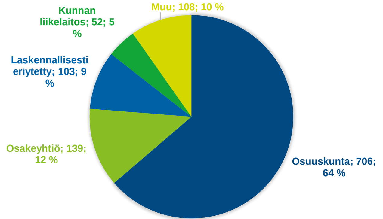
VESIHUOLTOLAITOSTEN TOIMINTAMUODOT
